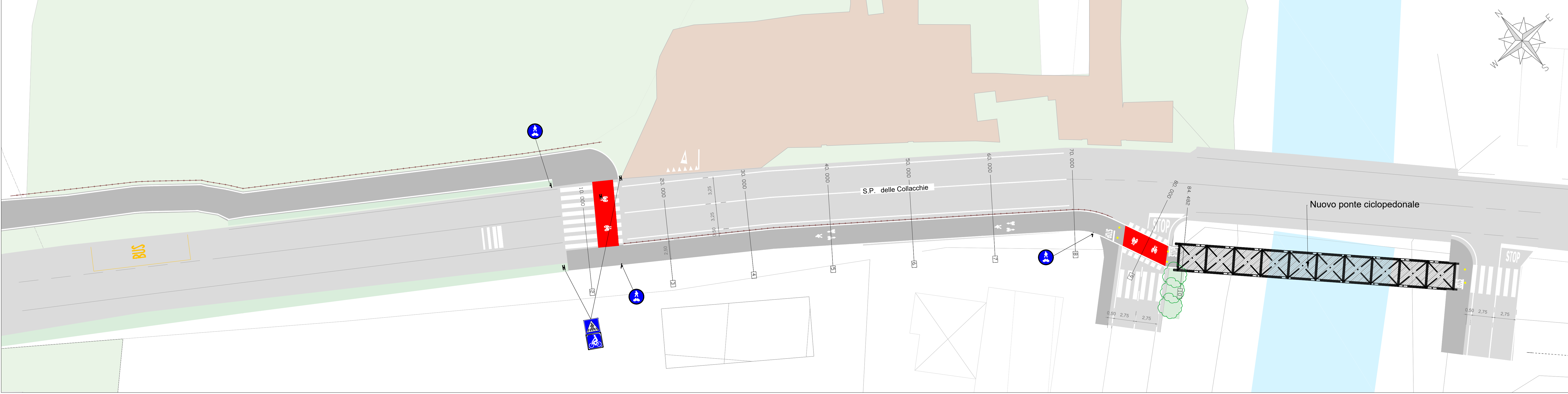
PLANIMETRIA PONTE CICLOPEDONALE Scala 1:100
