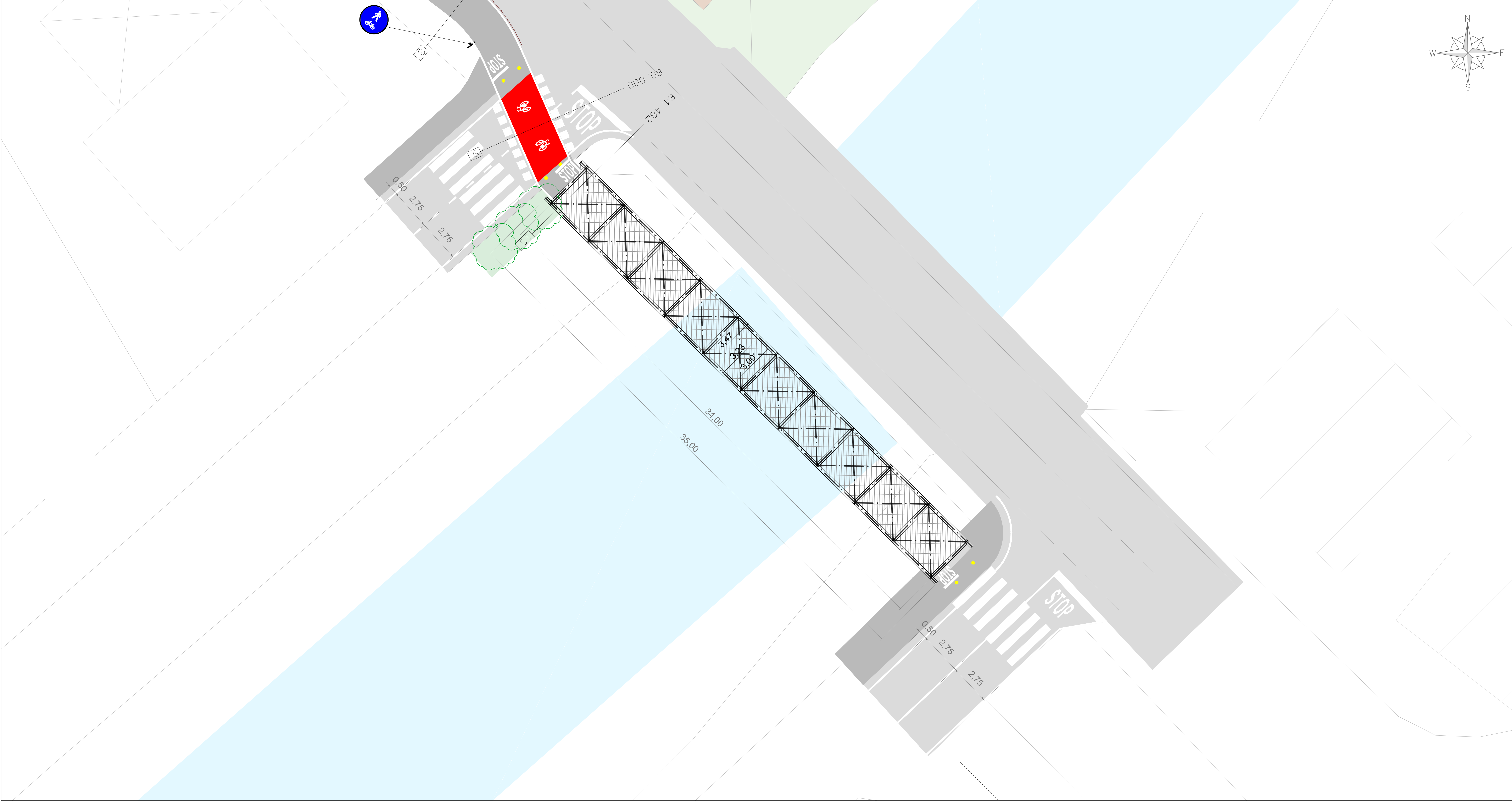
PLANIMETRIA PONTE CICLOPEDONALE Scala 1:100
